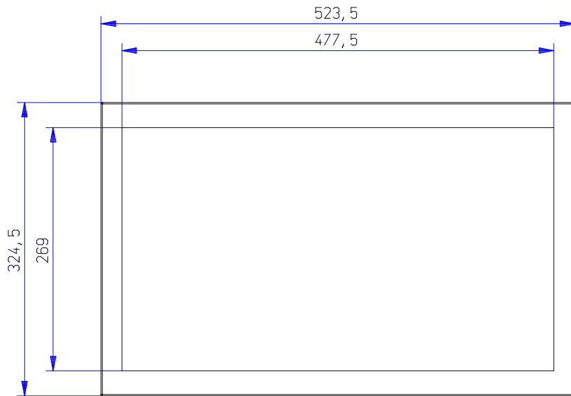
Frontansicht
