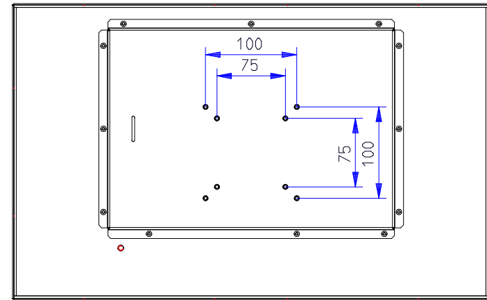
Rückansicht
